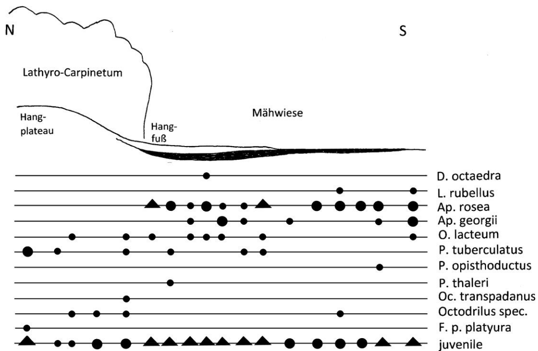
Abbildung 2. Regenwurmfauna der untersuchten Bodenstandorte im Hang-Transsekt bei Betfalva. Mit dunklem Horizont des Inversprofils. Die Punkte bzw. Dreiecke repräsentieren die Individuendichte der adulten Regenwürmer und der Juvenilen in drei Größenklassen: • 1-3, ● 4-10, ▲ >10 Individuen auf 0,25 m 2 untersuchter Fläche. Transektlänge ca. 80 m.
